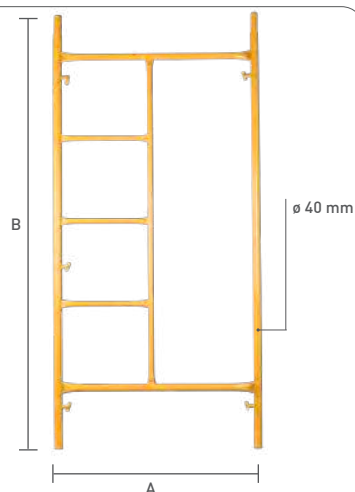
LATERAL DE ANDAIME 2mt PT MARCO DE ANDAMIO 2000mm LATÉRAL D'ÉCHAFAUDAGE 2000mm SCAFFOLDS SEITE 2000mm SIDE OF SCAFFOLD 2000mm
