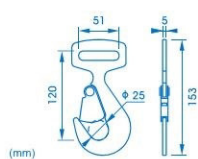
ref.ª GPS5000 gancho com patilha, 5000 kg flat snap hook, 5000 kg
