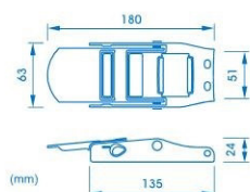
ref.ª TCZINC / TCINOX esticador de cortina zincado ou inox overcenter buckle zinc coated or stainless steel
