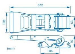
ref.ª T5T50I invertido, 5000 kg inverted, 5000 kg
