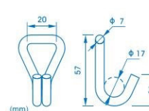
ref. o G1000J gancho em j, 1000 kg double j hook, 1000 kg
