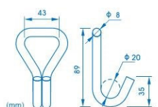
ref. o G2000J gancho em j, 2000 kg double j hook, 2000 kg
