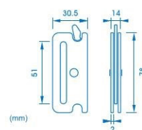
ref.º GF50 gancho frigoríficos end buckle
