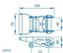
ref.ª T2T35 pega larga, 2000 kg wide handle, 2000 kg
