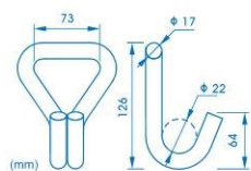
ref. o G10000J gancho em j, 10000 kg double j hook, 10000 kg
