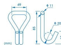
ref. o G5000J gancho em j, 5000 kg double j hook, 5000 kg
