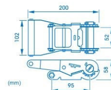
ref.ª T5T50 pega média, 5000 kg medium handle, 5000 kg
