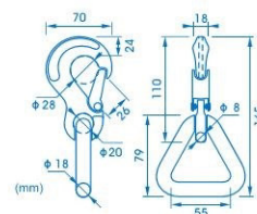
ref.ª G5PES5000 gancho c/ argola em triangulo, 5000 kg forged hook with triangle ring, 5000 kg
