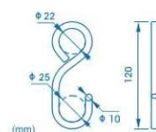
ref.ª G10008 gancho em s, 1000 kg s hook, 1000 kg
