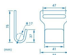
ref.ª GCHAPAN gancho em chapa flat hook
