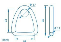
ref.ª G5000D argola em d, 5000 kg d ring, 5000 kg
