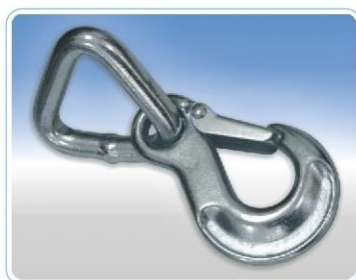
ref.ª G5PES5000 gancho c/ argola em triangulo, 5000 kg forged hook with triangle ring, 5000 kg
