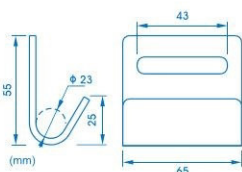
ref.ª GCHAPA gancho em chapa flat hook
