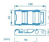
ref.ª TFM esticador de cortina overcenter buckle
