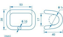
ref.ª GARAME gancho em arame close rave hook
