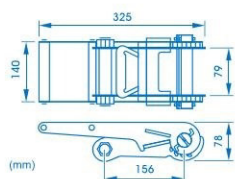
ref.ª T10T75 pega comprida, 10000 kg long handle, 10000 kg
